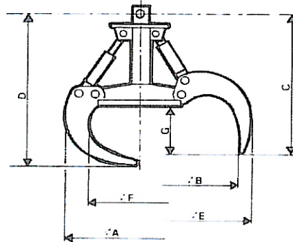
GIRO CONTROLADO CON MOTOR HIDRÁULICO
